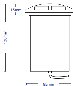
INGRESS IP66
